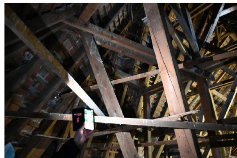
Innenhöhe begrenzt mit Kükendraht, Dachlatten zum Absitzen von Tauben, Giebelnischen mit Brettern
