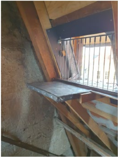
Projektsicherheit: Pendeleinflug gegen Eindringen von Greifvögeln im Taubeneinflug erstellt.
